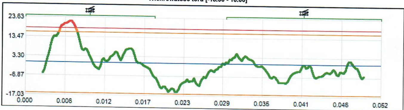
Wichrowatość toru [-18.00 - 18.00]
